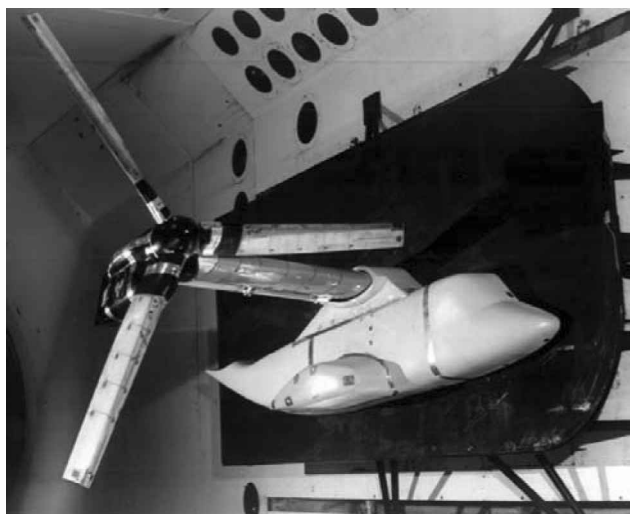
Fig. 16 WRATS tilt-rotor testbed in the TDT.
